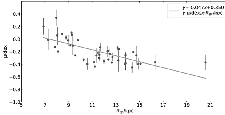
图 3 老年疏散星团样本给出的银盘金属丰度径向轮廓, 横坐标是银心距, 纵坐标是 [\text{Fe}/\text{H}] 的平均值 \mu , 图中散点是样本中老年疏散星团的观测值, 直线是用最小二乘法拟合的结果.
